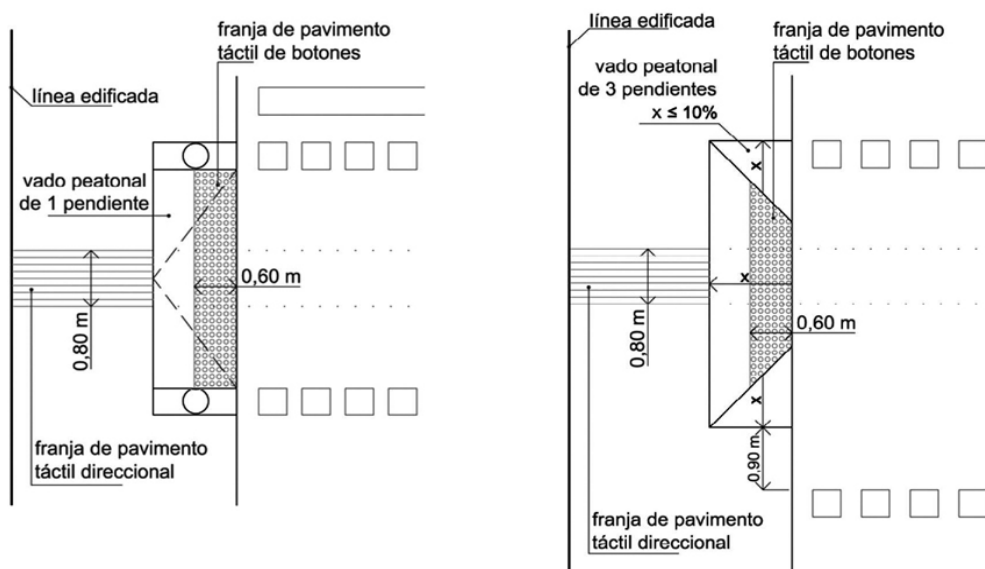
Figura 1: Pas peatonal d'una i tres pendents.
