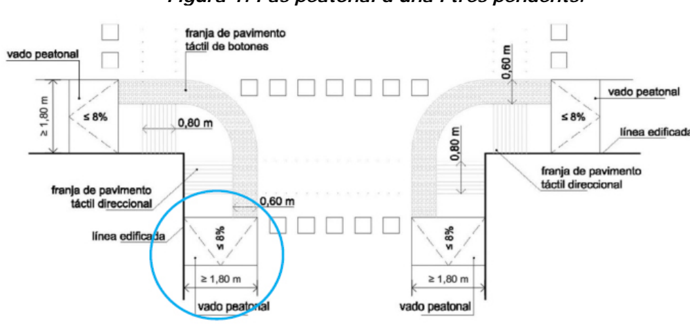
Figura 2: Pas peatonal amb rebaixament horitzontal.
